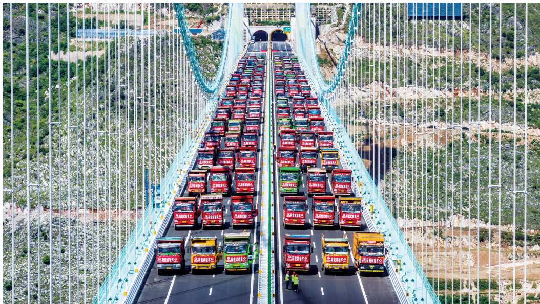
2025年8月25日拍摄的贵州花江峡谷大桥荷载试验现场（无人机照片）。（新华社发）
